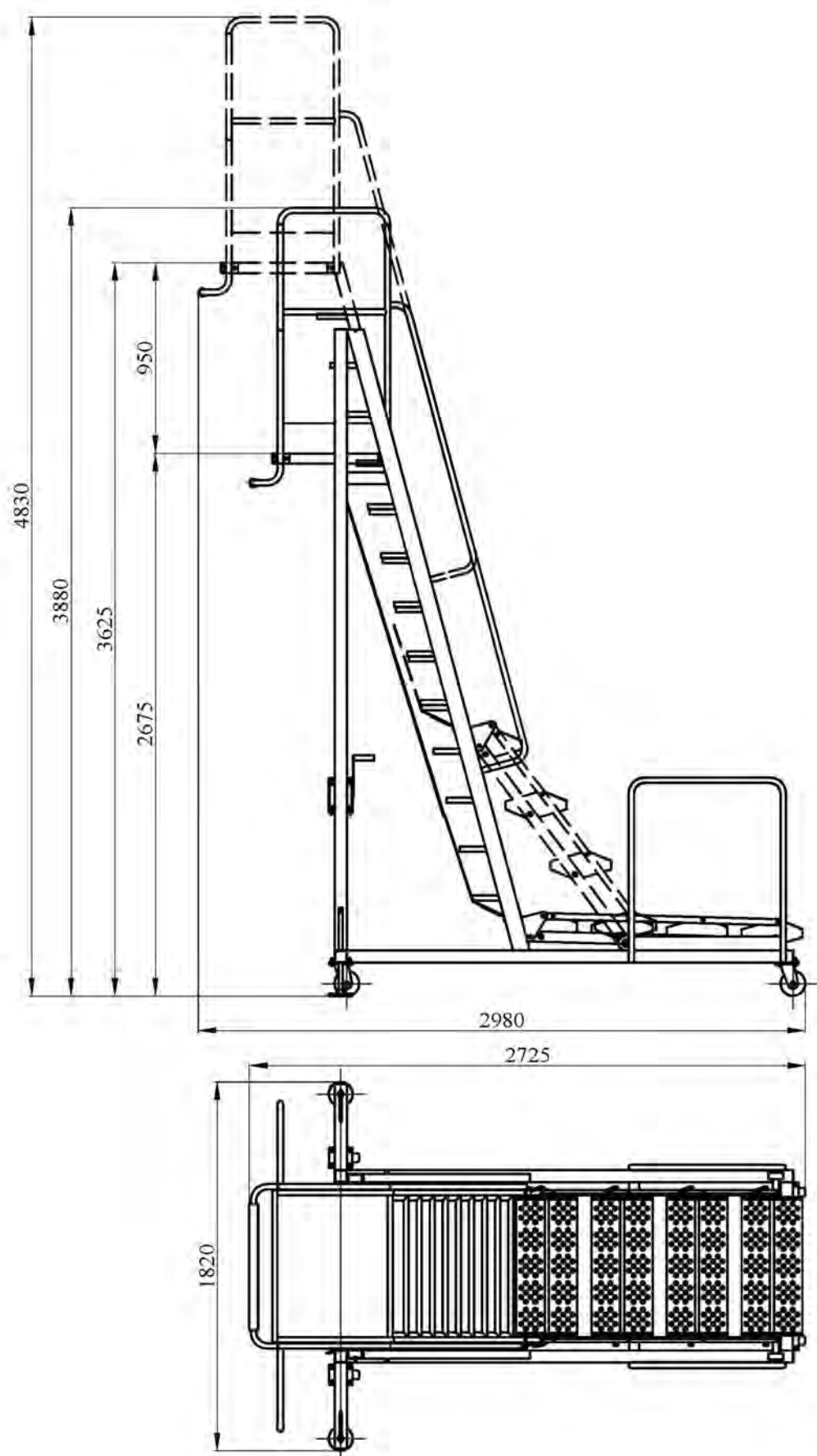
Рисунок 2 - Основные размеры площадки ПО-13
