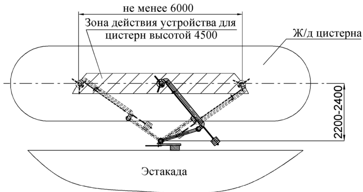
Рисунок 7а- Зона действия устройства
