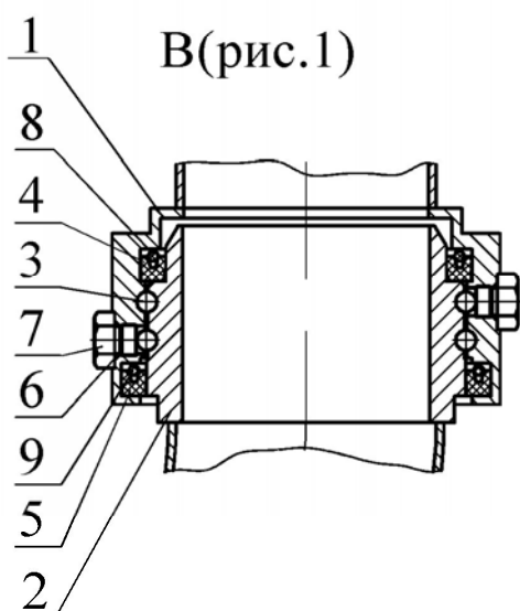
Рисунок 4-Шарнир соединительный
