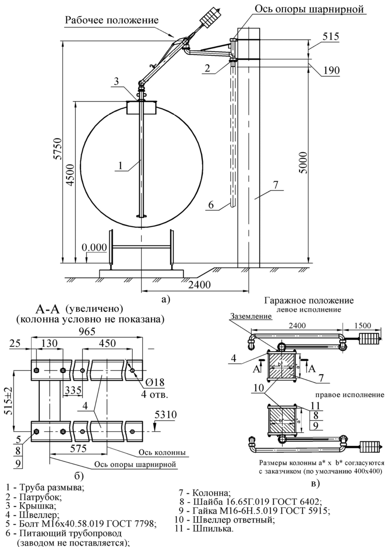
Рисунок 6-Монтажная схема
