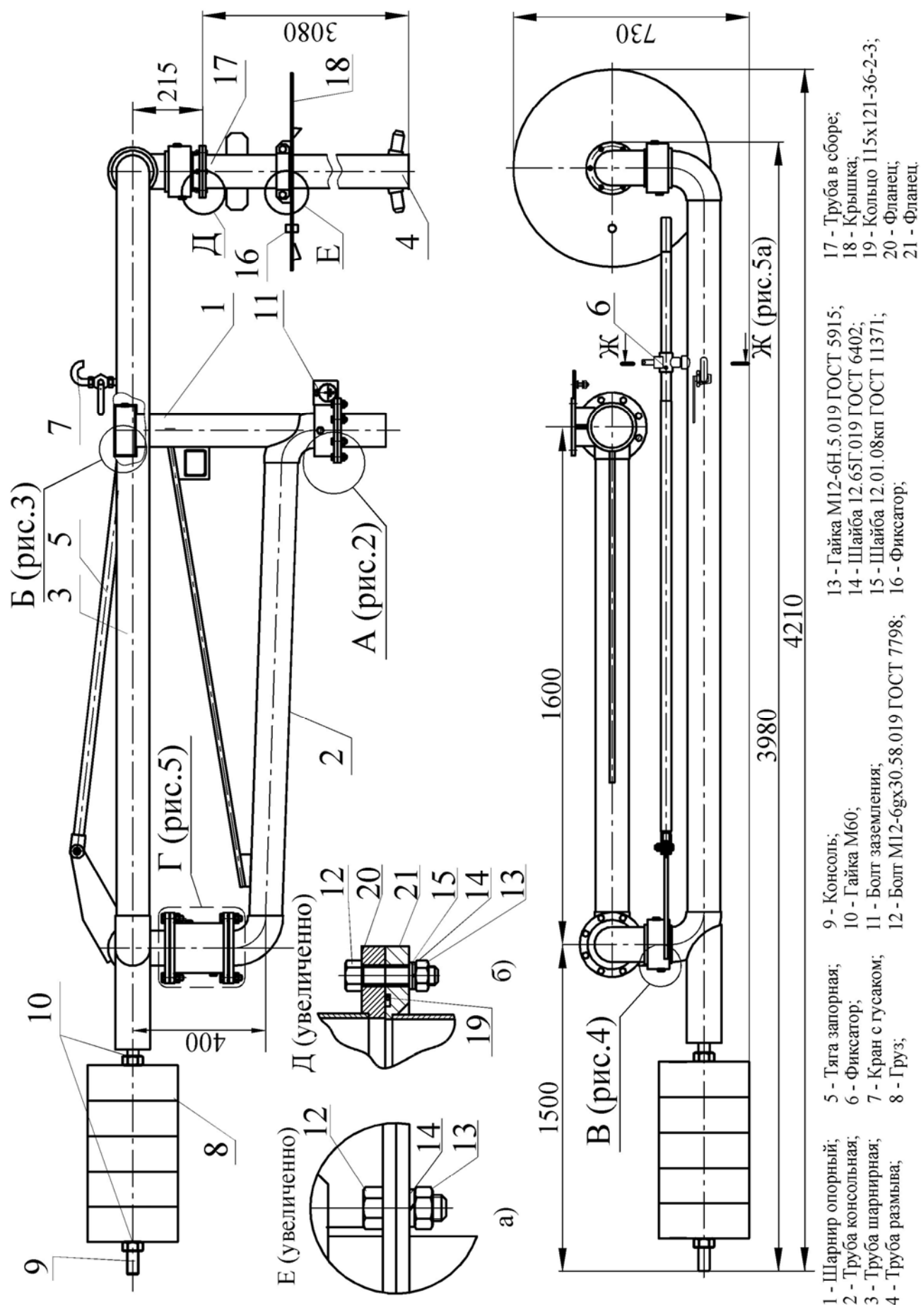
Рисунок 1-Общий вид устройства без системы управления наливом
